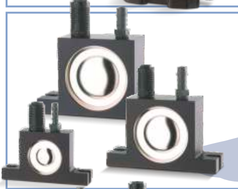
NCB Pnömatik Bilyalı Vibratörler
